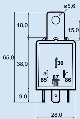
FASTON 6,3x0,8 ISO 8092 - 1
